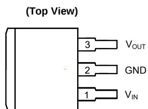
TO-263-3
